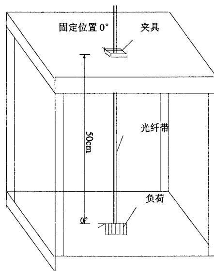
图 4 残余扭转试验装置
