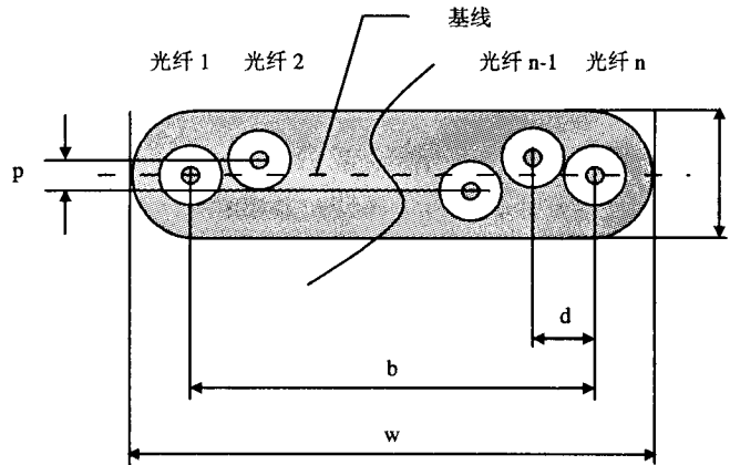
图 1 光纤带几何结构的横截面
